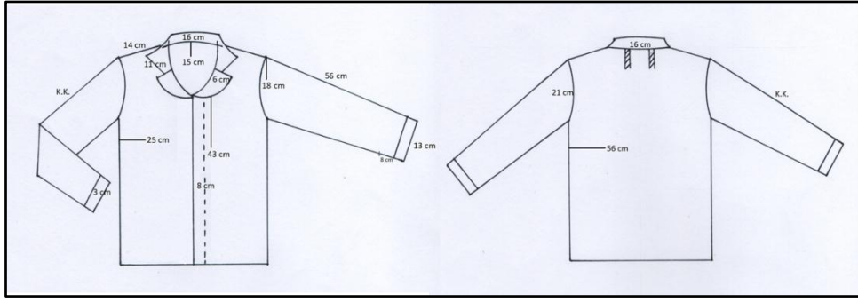
Çizim No: 2(Gömlek Ön-Arka)
